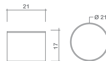
Side Top
